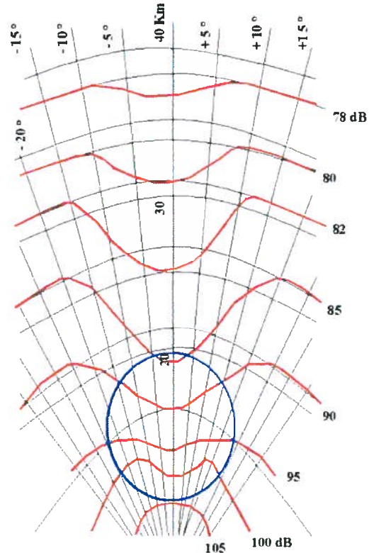
Fig. 3 - andamento delle linee di equal cmap e.m. basati sulle misure (Milano Siziano, 1035 MHz)
