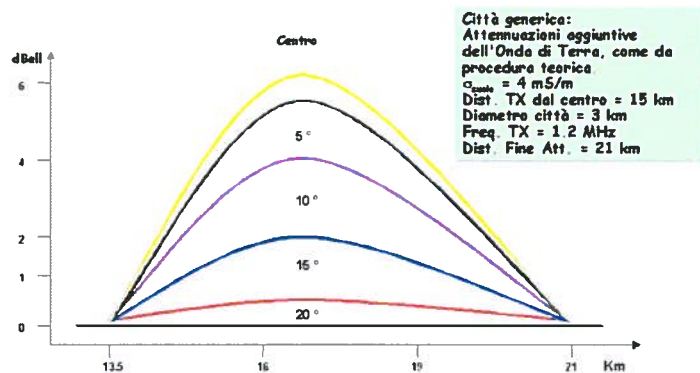
Fig. 8 - Città generica: Attenuazioni aggiuntive dell'Onda di Terra, come da procedura teorica. \sigma_{\text{suolo}} = 4 \text{ mS/m} Dist. TX dal centro = 15 km Diametro città = 3 km Freq. TX = 1.2 MHz Dist. Fine Att. = 21 km
