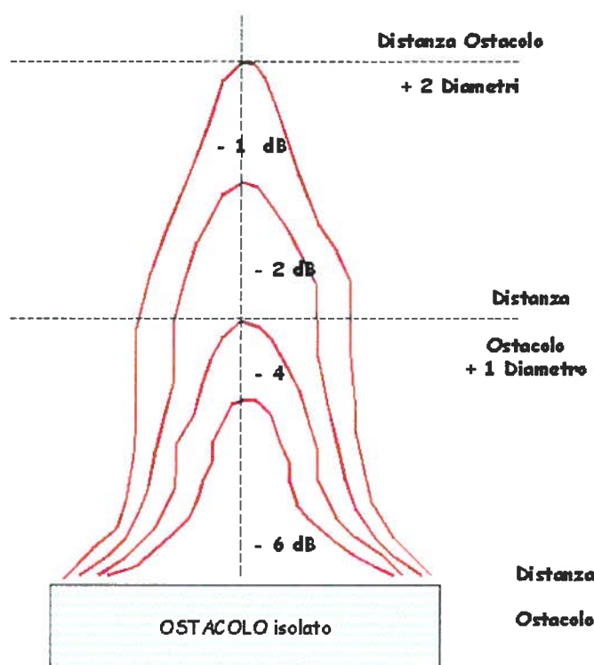
Fig. 9 - Tipiche attenuazioni dovute ad un ostacolo isolato tra due linee isocampo
