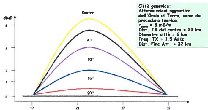
Fig. 7 - Città generica: Attenuazioni aggiuntive dell'Onda di Terra, come da procedura teorica. \sigma_{\text{suolo}} = 8 \text{ mS/m} Dist. TX dal centro = 20 km Diametro città = 6 km Freq. TX = 1.5 MHz Dist. Fine Att. = 32 km
