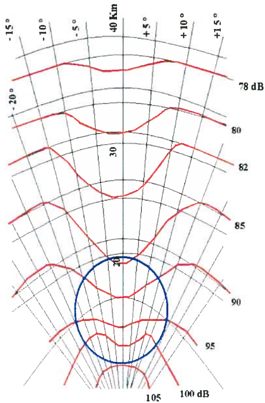
Fig. 2 - andamento delle linee di equal cmap e.m. basati sulle misure (Milano Siziano, 900 MHz)
